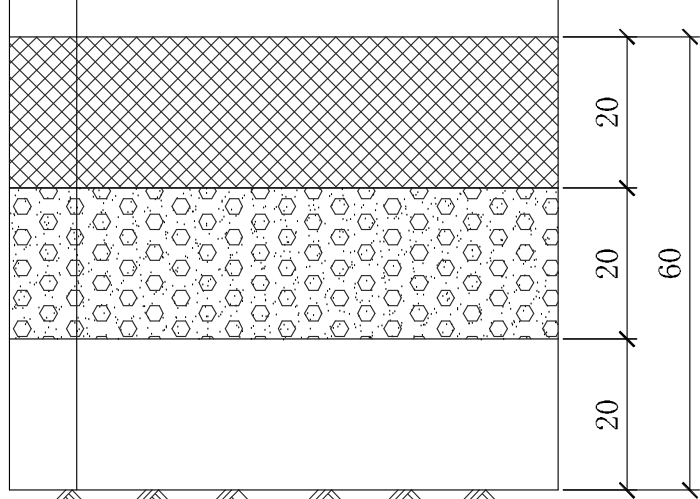
水泥混凝土道路结构图
